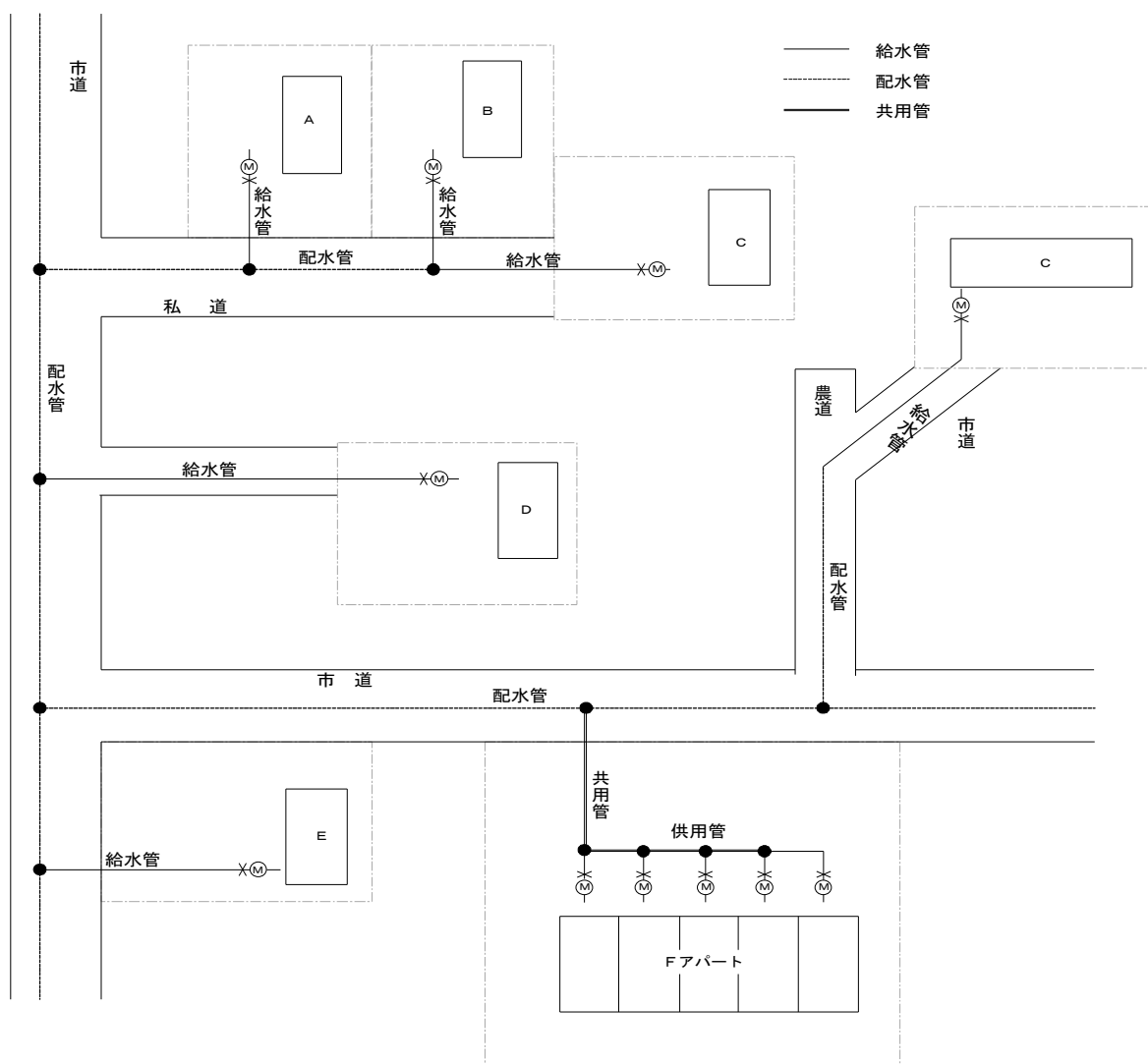
図(配水・給水・共用管区分図)
